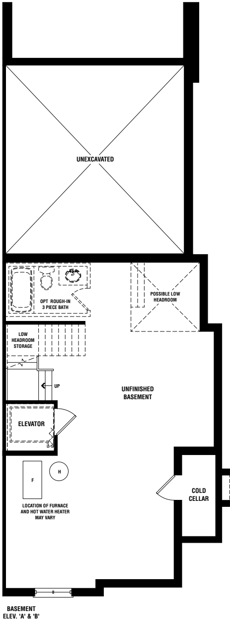
BASEMENT ELEV. 'A' & 'B'
